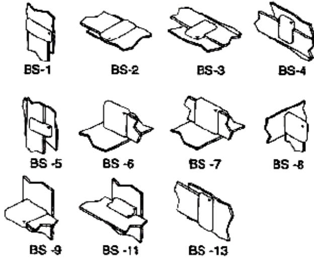
LUG OR BUS BAR TO STEEL
