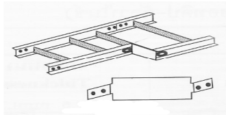
L-CS-001 ข้อลดความกว้าง
