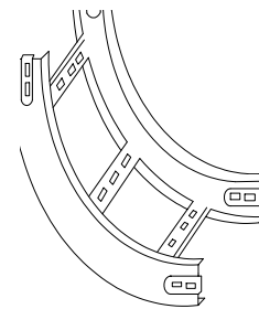
งอขึ้นแลดเดอร์ (INSIDE VERTICAL RISER)
