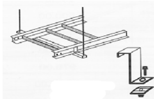
L-CS-006 แคลมป์ยึดเพดาน HOLD DOWN CLAMP
