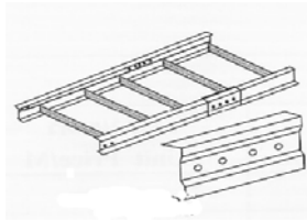
L-CS-005 ข้อต่อตรง SPLICE PLATE
